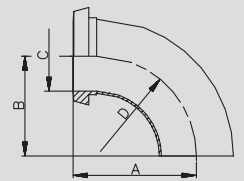
Bogen KK DIN 90° bend liner/liner DIN 90°
